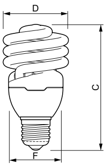
TORNADO 23W CDL E27 110-127V 50/60Hz
