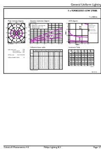
LEDbulb CLA 4,5W G16,5 E27 827
