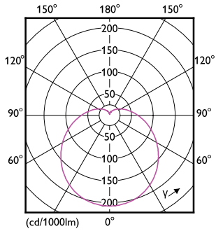
LEDbulb 9W A60 E27 830 FR
