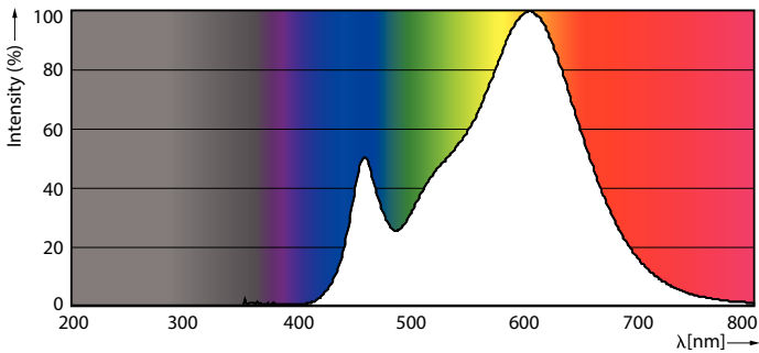
LEDbulb 9W A60 E27 830 FR
