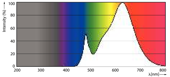
Spectral Power Distribution Colour - 14A19/LED/830/FR/P/ND 1PF/6 NL
