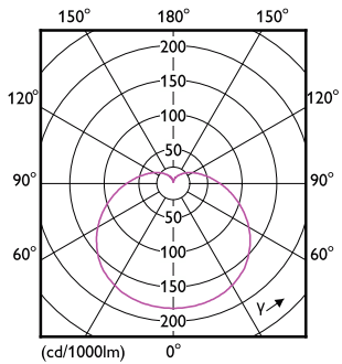
Light Distribution Diagram - 14A19/LED/830/FR/P/ND 1PF/6 NL
