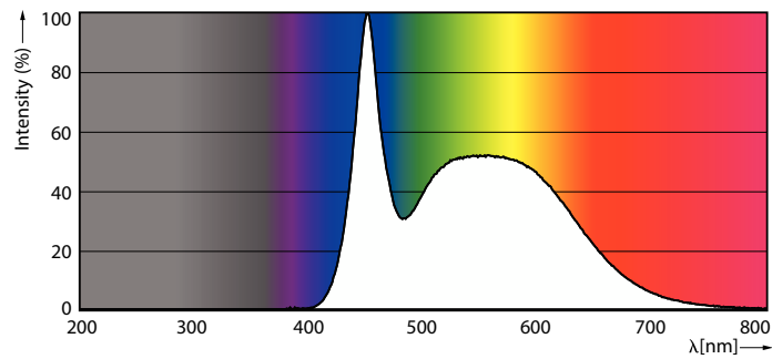
Spectral Power Distribution Colour - 11A19/LED/865/FR/P/ND 1PF/6 NL
