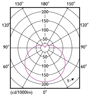
Light Distribution Diagram - 11A19/LED/865/FR/P/ND 1PF/6 NL
