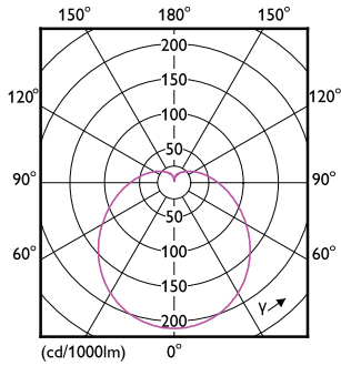
Light Distribution Diagram - 6A19/LED/865/FR/P/ND 2PF/6 NL
